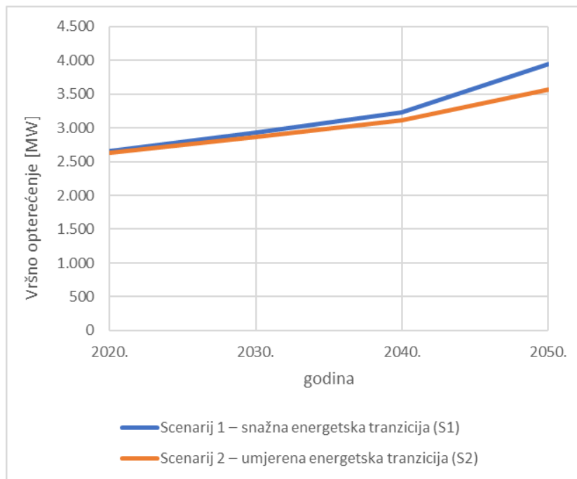
Slika 10.15. Vršno opterećenje za razini distribucijske mreže (vrednovan utjecaj distribuiranih izvora priključenih na distribucijsku mrežu)
