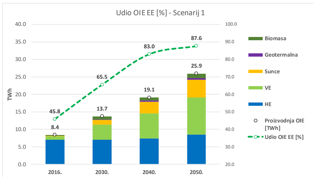
Slika 10.54. Udio OIE u proizvodnji električne energije – Scenarij 1
