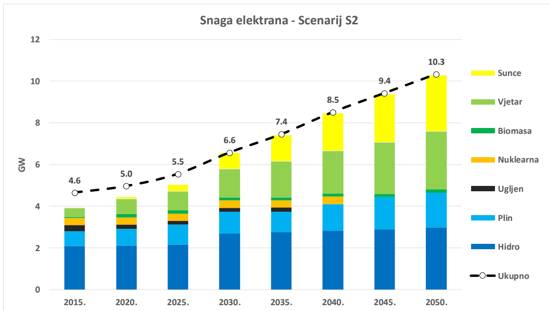
Slika 10.35. Snaga elektrana do 2050. godine – Scenarij 2
