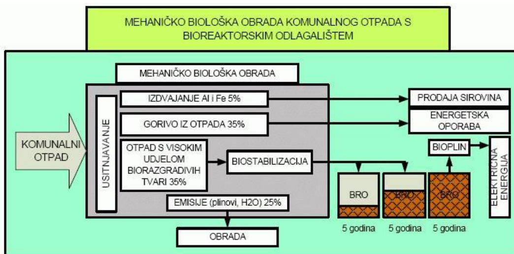
Slika 8.7. Shema procesa mehaničko-biološke obrade komunalnog otpada 191
