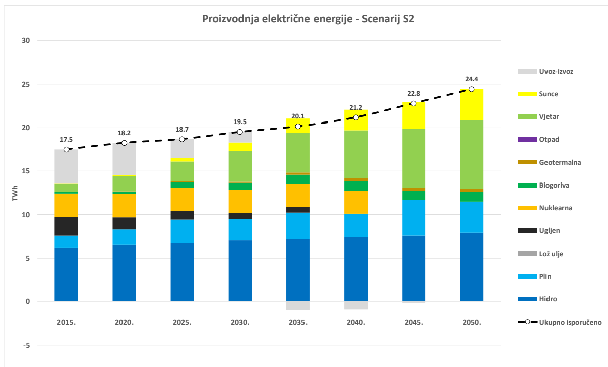
Slika 10.37. Proizvodnja električne energije – Scenarij 2
