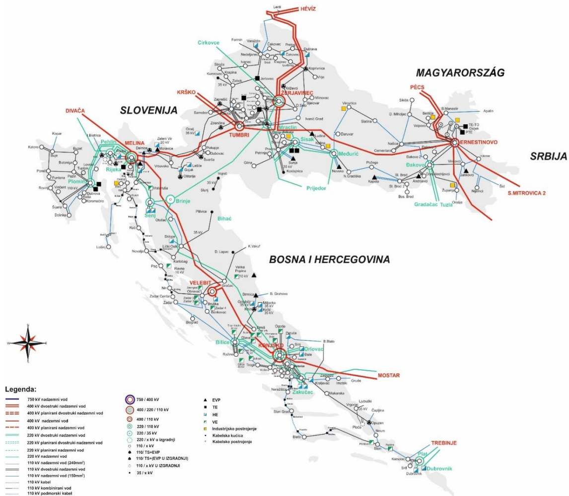
Slika 3.30. Hrvatska prijenosna elektroenergetska mreža
