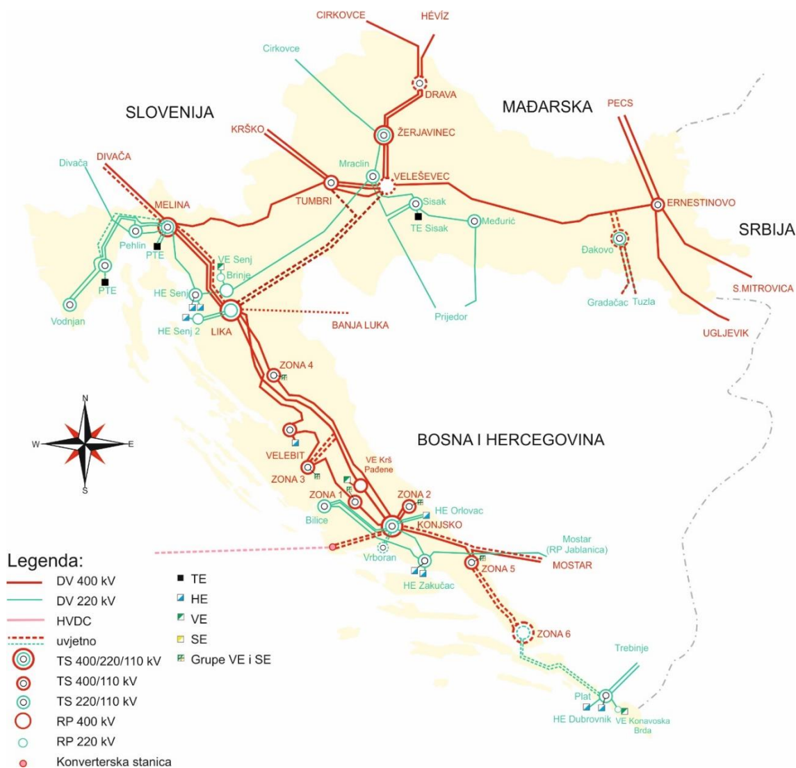
Slika 10.14. Skica predvidive topologije 400 kV i 220 kV mreže na području RH 2050. godine
