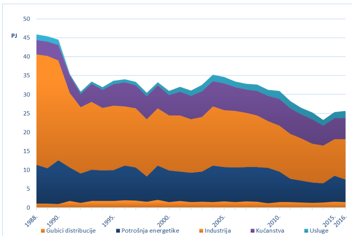
Slika 3.40. Potrošnja toplinske energije u Hrvatskoj
