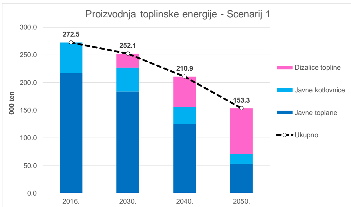
Slika 10.27. Proizvodnja toplinske energije – Scenarij 1
