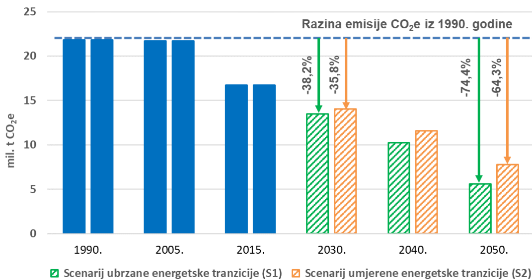
Slika 11.3. Projekcija ukupnih emisija stakleničkih plinova za Scenarij 1 i Scenarij 2
