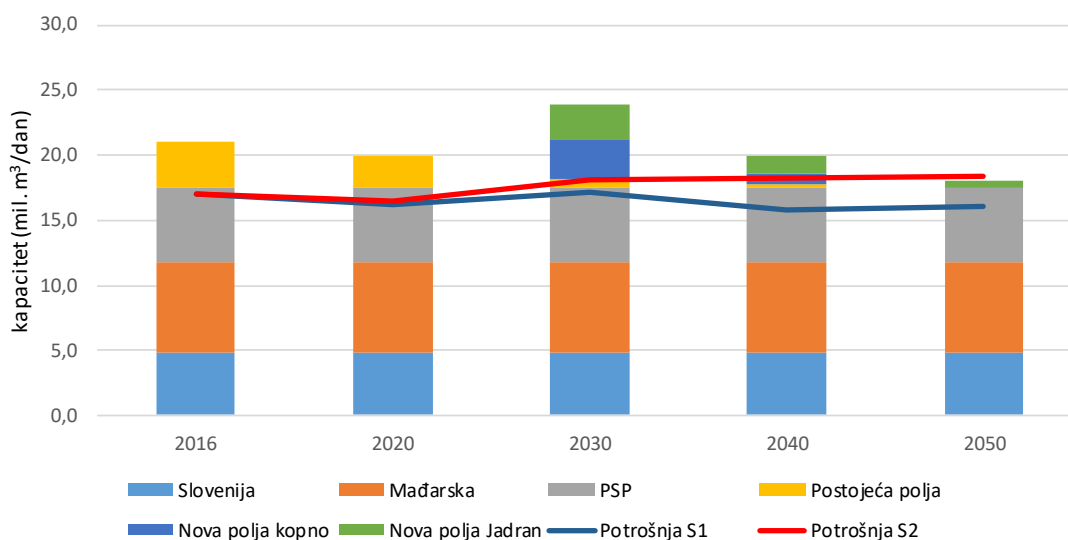
Slika 10.22. Kapaciteti opskrbe i vršna potrošnja plina kod iznimno hladne zime
