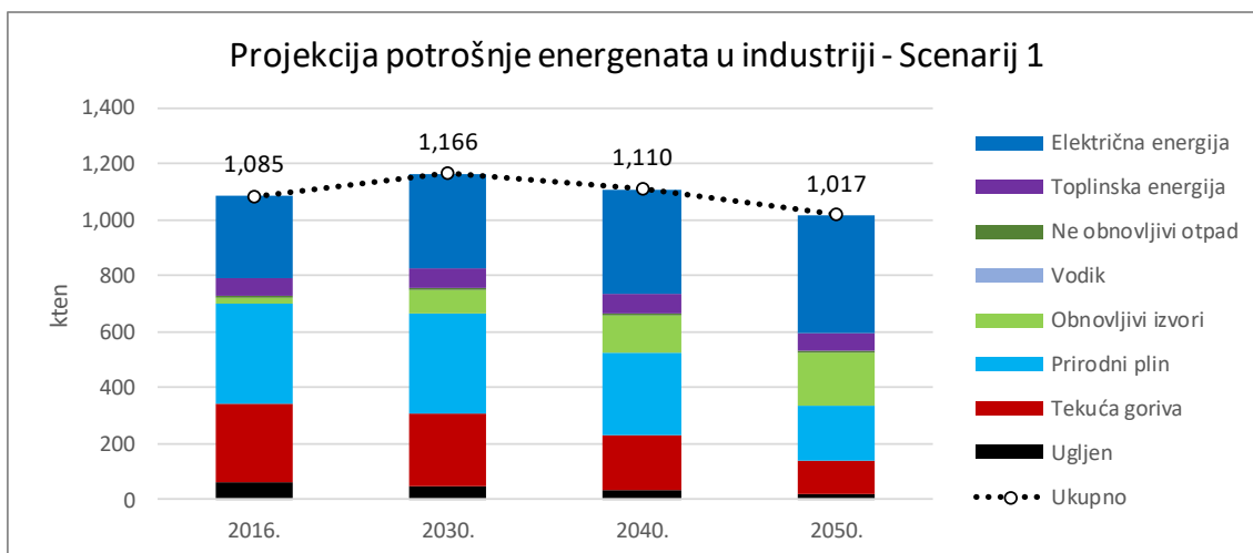
Slika 10.4. Projekcija potrošnje energenata u industriji (Scenarij 1)
