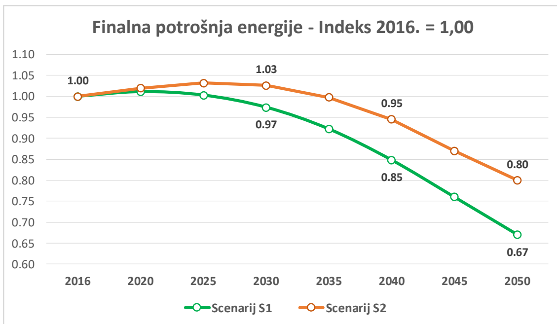
Slika 10.49. Finalna potrošnja energije – promjena u odnosu na 2016. godinu – Scenarij 1 i Scenarij 2
