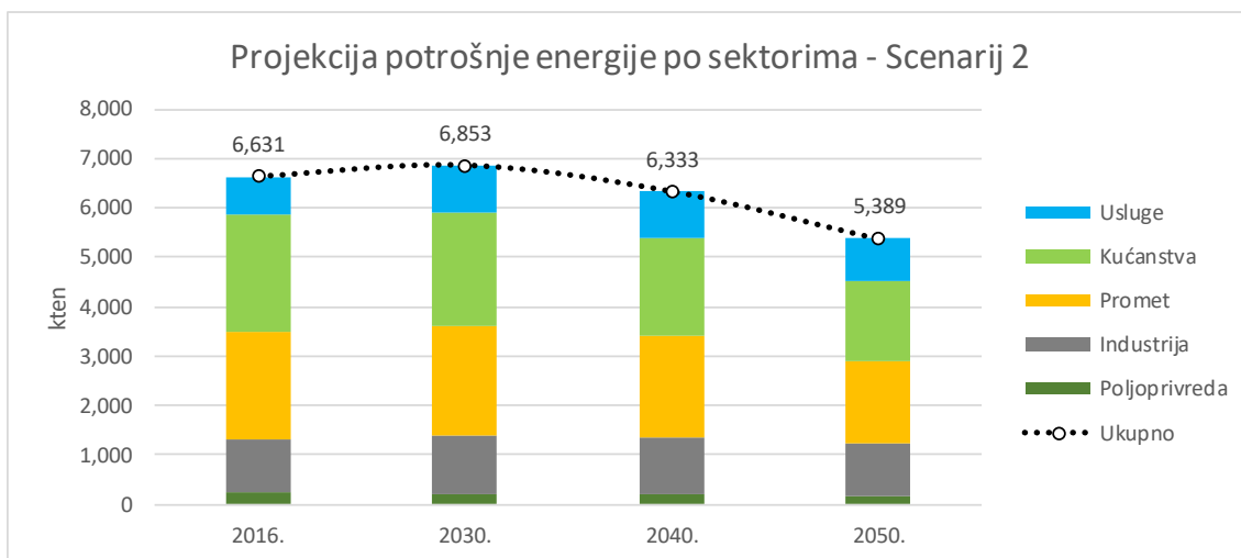
Slika 10.29. Projekcija potrošnje energije po sektorima (Scenarij 2)
