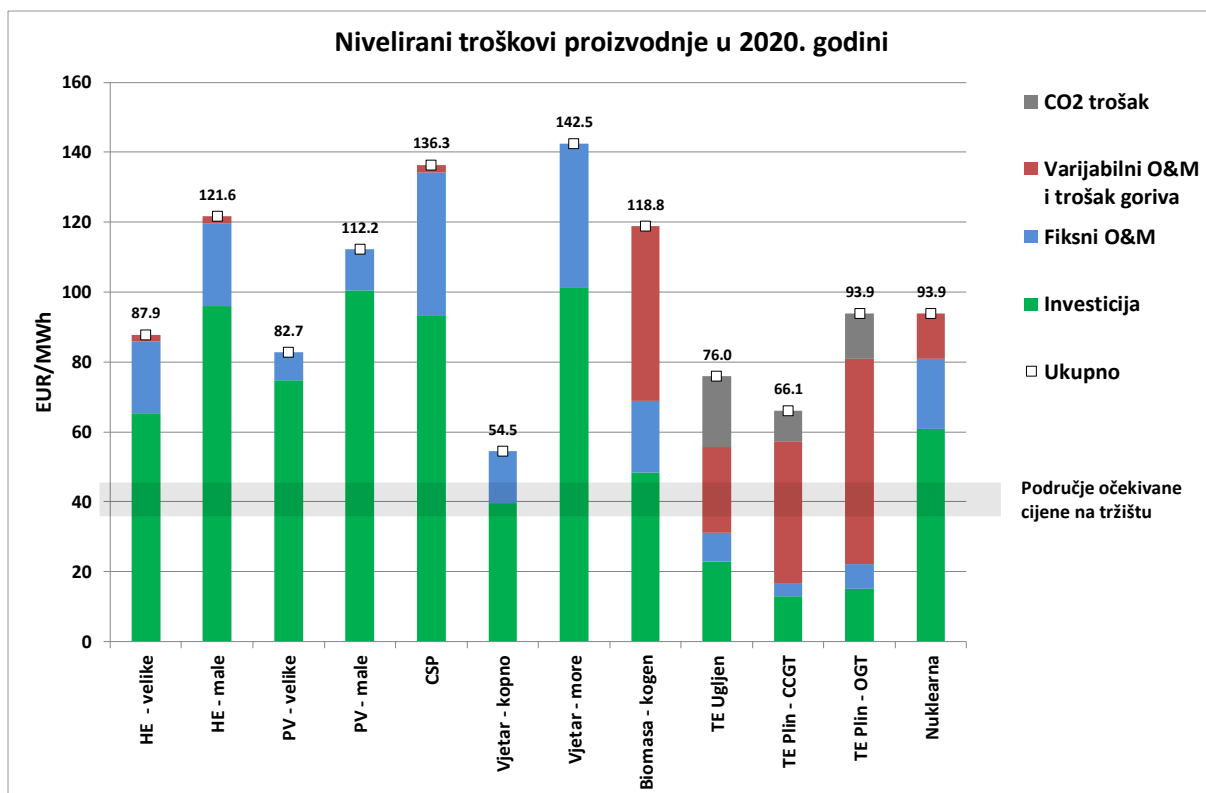
Slika 8.18. Nivelirani troškovi proizvodnje električne energije u 2020. godini
