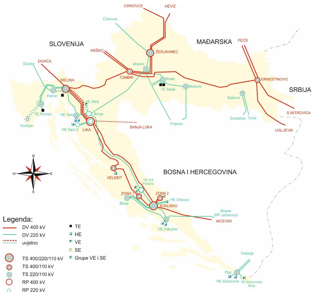
Slika 10.13. Predvidiva topologija 400 kV i 220 kV mreže na području RH 2030. godine
