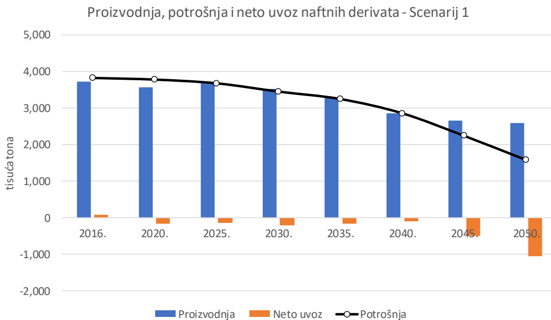
Slika 10.17. Projekcija proizvodnje, potrošnje i neto uvoza naftnih derivata (Scenarij 1)
