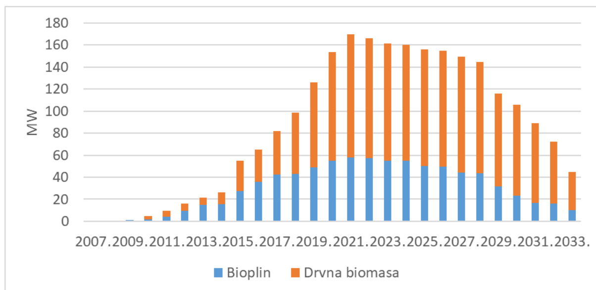
Slika 3.16. Procjena kapaciteta proizvodnje električne energije iz drvene biomase i bioplina u Hrvatskoj 68
