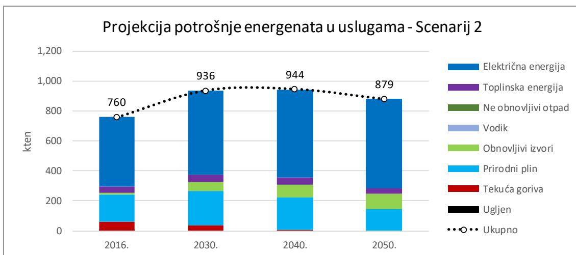
Slika 10.34. Projekcija potrošnje energenata u uslugama (Scenarij 2)
