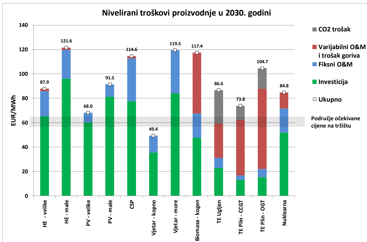
Slika 8.19. Nivelirani troškovi proizvodnje električne energije u 2030. godini
