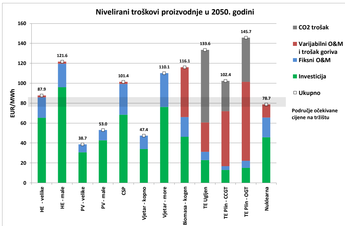
Slika 8.20. Nivelirani troškovi proizvodnje električne energije u 2050. godini
