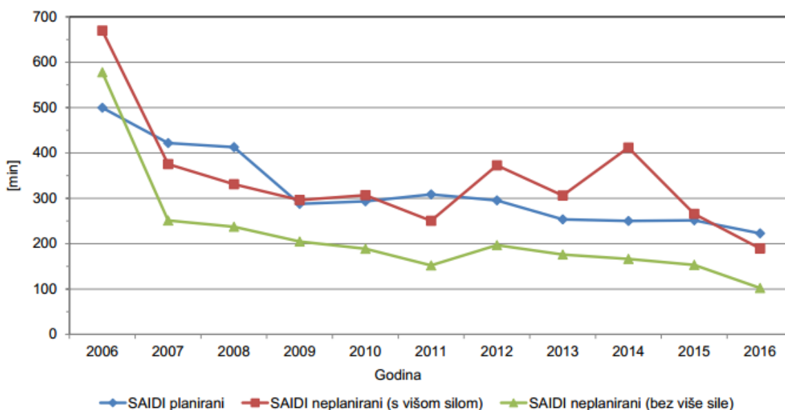
Slika 3.33. Prosječno trajanje dugotrajnih prekida napajanja po korisniku mreže (SAIDI) u razdoblju 2007. - 2016.
