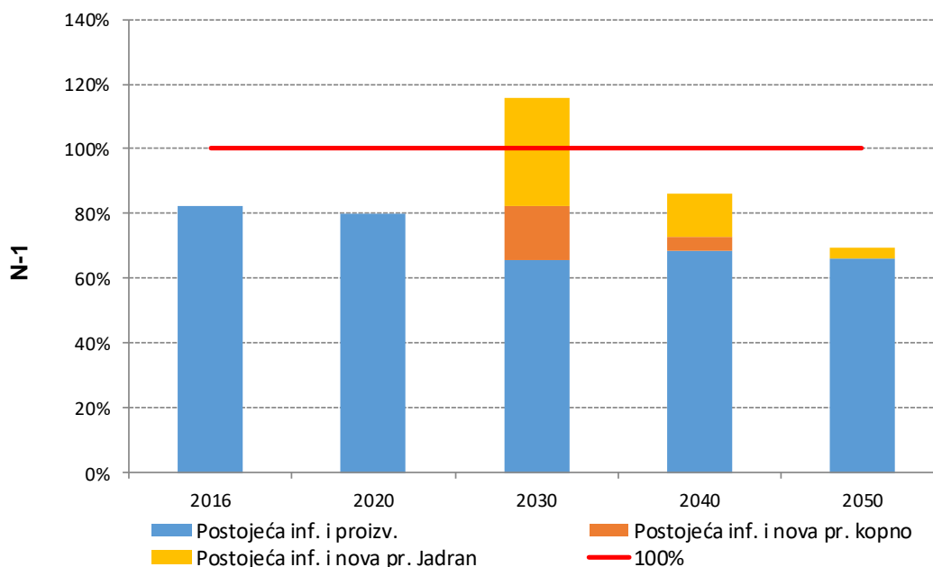
Slika 10.24. Pokazatelj N-1 za scenarij potrošnje S1
