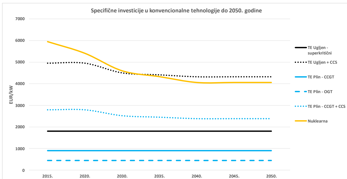
Slika 8.17. Specifična investicija u elektrane na fosilna goriva i nuklearne elektrane
