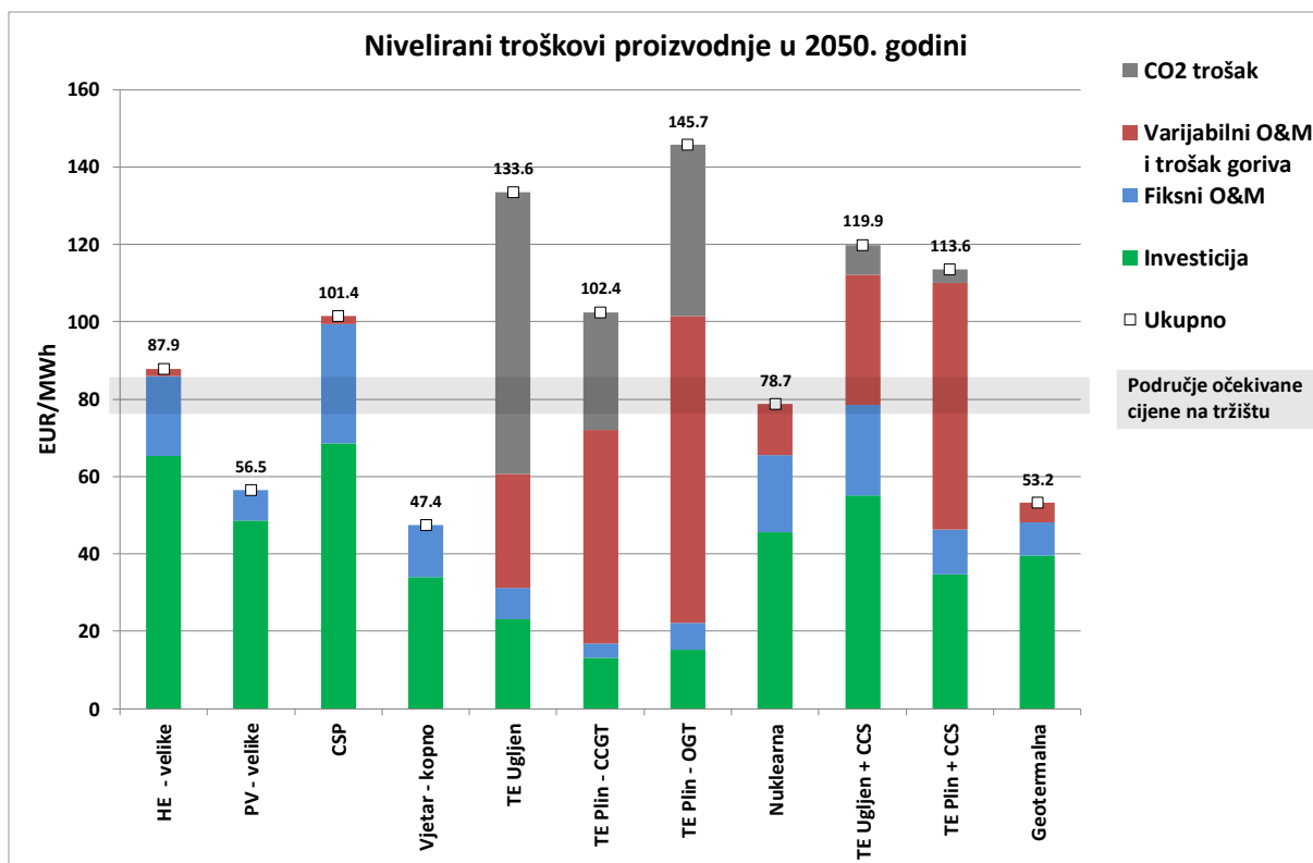
Slika 8.21. Nivelirani troškovi proizvodnje električne energije u 2050. godini
