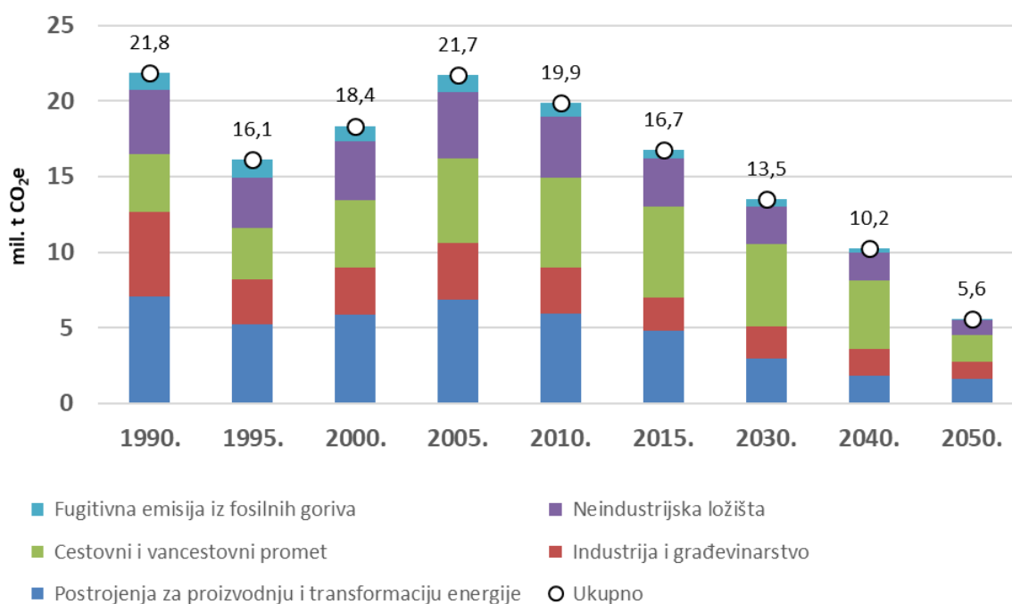
Slika 11.1. Projekcija emisija stakleničkih plinova prema Scenariju 1
