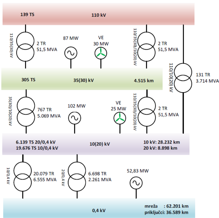
Slika 3.31. Osnovni podaci o distribucijskom sustavu na dan 31. prosinca 2017. godine
