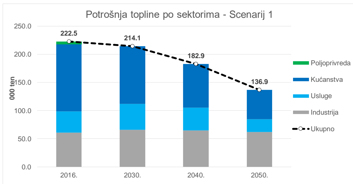
Slika 10.26. Finalna potrošnja toplinske energije po sektorima potrošnje – Scenarij 1
