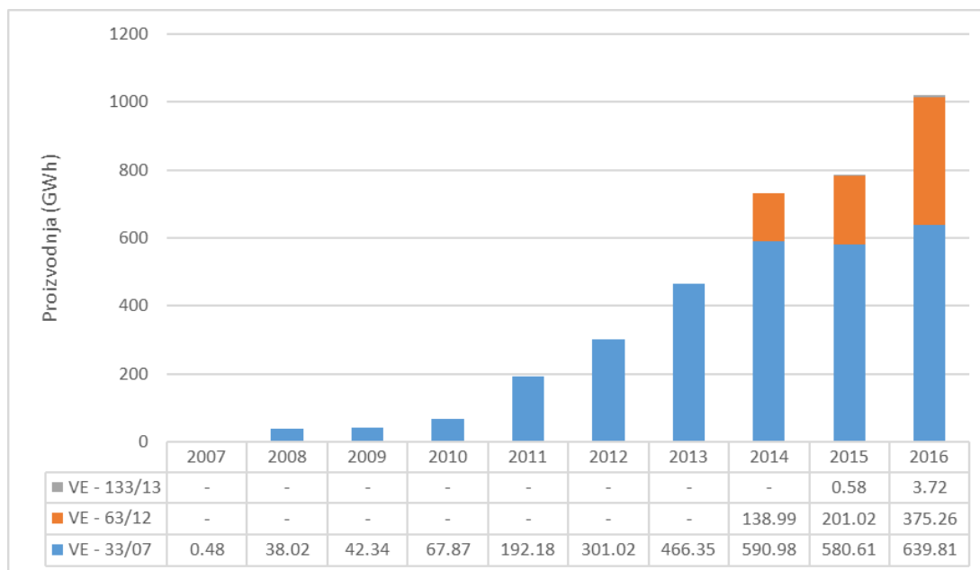
Slika 3.6. Godišnja proizvodnja iz vjetroelektrana u razdoblju 2007.-2016. godine
