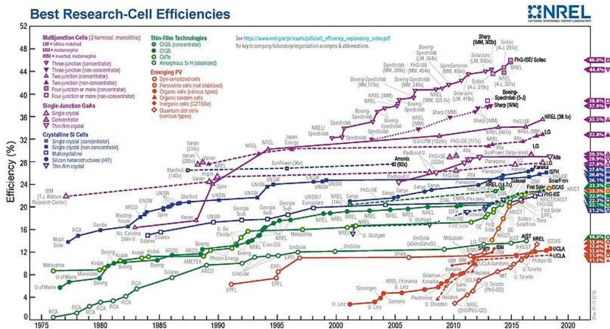
Slika 8.14. Kretanje postignutih učinkovitosti sunčanih ćelija
