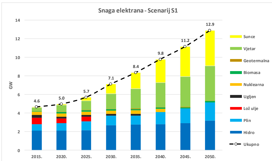
Slika 10.8. Snaga elektrana do 2050. godine – Scenarij 1
