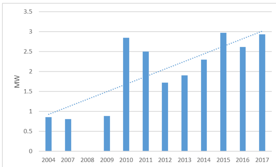
Slika 8.12. Trend jedinične snage vjetroagregata u Republici Hrvatskoj
