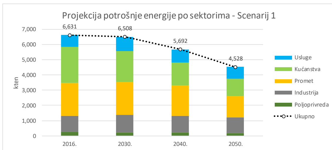
Slika 10.1. Projekcija potrošnje energije po sektorima (Scenarij 1)
