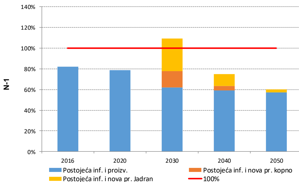
Slika 10.44. Pokazatelj N-1 za potrošnju prema Scenariju 2
