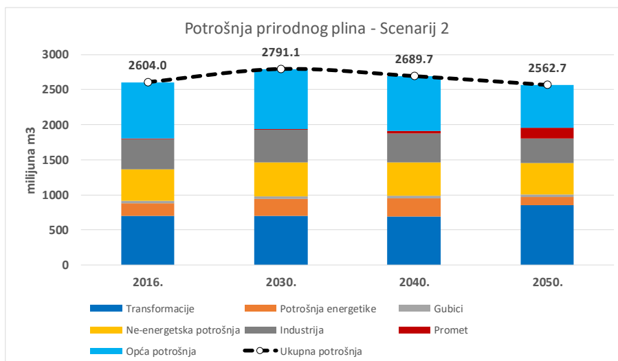
Slika 10.43. Potrošnja i proizvodnja prirodnog plina – Scenarij 2
