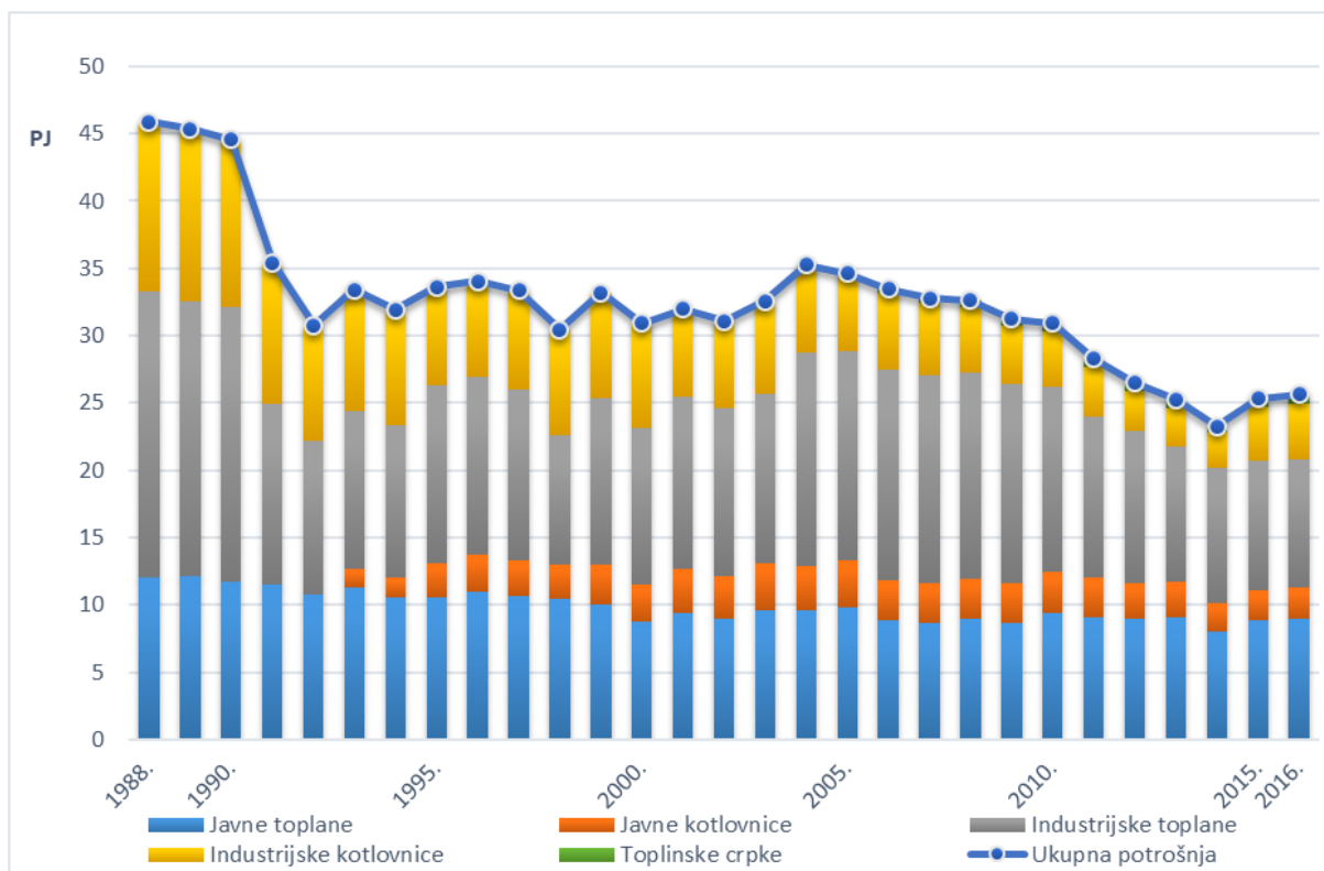
Slika 3.39. Proizvodnja toplinske energije u Hrvatskoj od 1988. do 2016. godine
