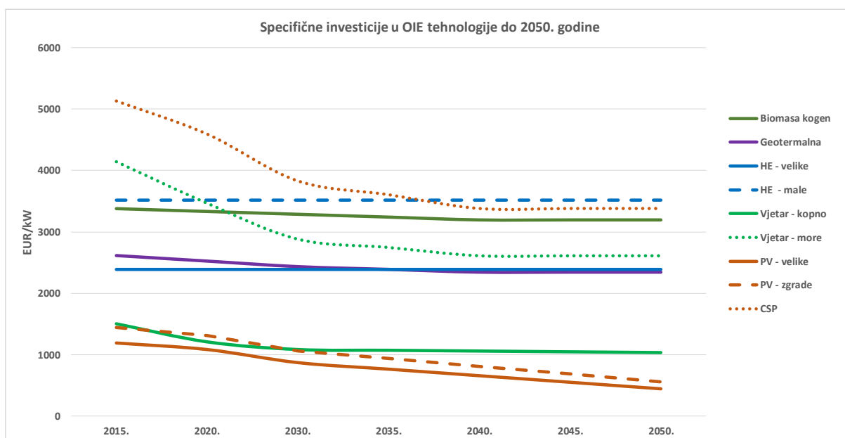
Slika 8.16. Specifična investicija u OIE tehnologije
