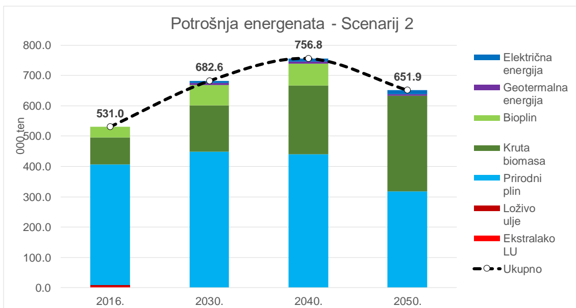
Slika 10.47. Potrošnja energenata za proizvodnju toplinske i električne energije u javnim toplanama, javnim kotlovnicama i dizalicama topline
