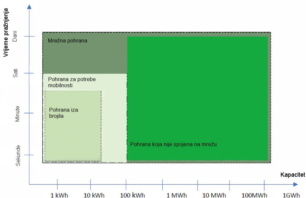
Slika 8.15. Tipični kapaciteti sustava pohrane energije
