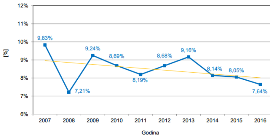
Slika 3.32. Gubici električne energije u distribucijskoj mreži u razdoblju 2007. - 2016.
