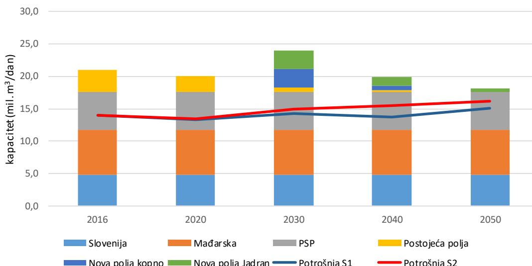
Slika 10.21. Kapaciteti opskrbe i vršna potrošnja plina kod prosječne zime
