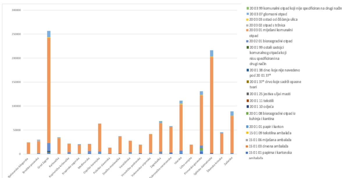
Slika 3.23. Biorazgradiva komponenta komunalnog otpada prema prijavljenim podacima za 2016. godinu po županijama u Republici Hrvatskoj 99
