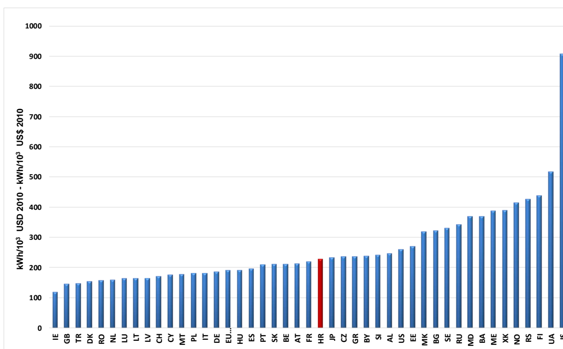
Slika 3.45. Intenzivnost bruto potrošnje električne energije prema paritetu kupovne moći
