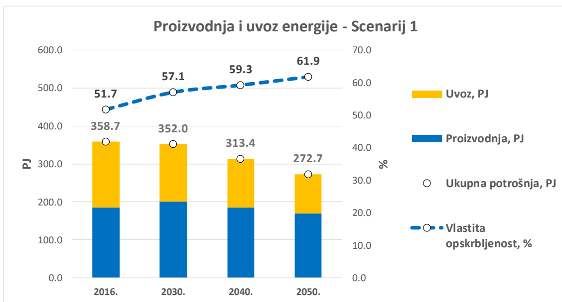
Slika 10.50. Vlastita opskrbljenost energijom – Scenarij 1
