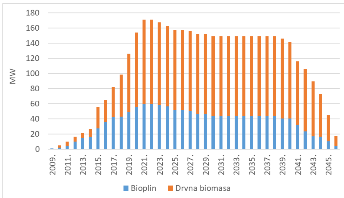
Slika 3.17. Procjena proizvodnih kapaciteta električne energije iz drvene biomase i bioplina 69
