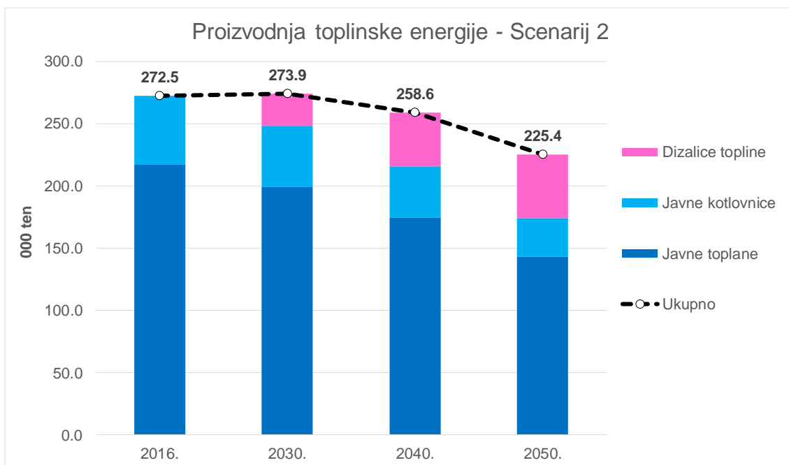
Slika 10.46. Proizvodnja toplinske energije – Scenarij 2
